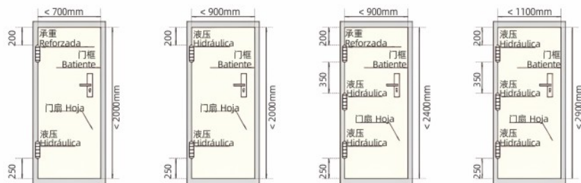
各门类定位功能示意图 Esquema de principio de la función de posicionamiento de cada segmento de puerta
