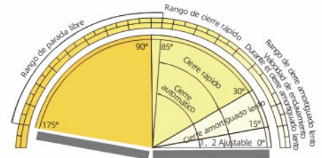
Esquema de principio de la función de posicionamiento de cada segmento de puerta
