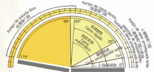
各门类定位功能示意图 Esquema de principio de la función de posicionamiento de cada segmento de puerta
