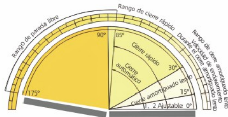
Esquema de principio de la función de posicionamiento de cada segmento de puerta
