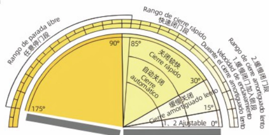
各门类定位功能示意图 Esquema de principio de la función de posicionamiento de cada segmento de puerta
